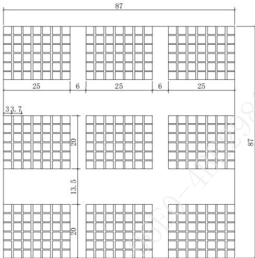
环氧树脂玻璃钢鱼礁单位鱼礁布局示意图（单位 m）
