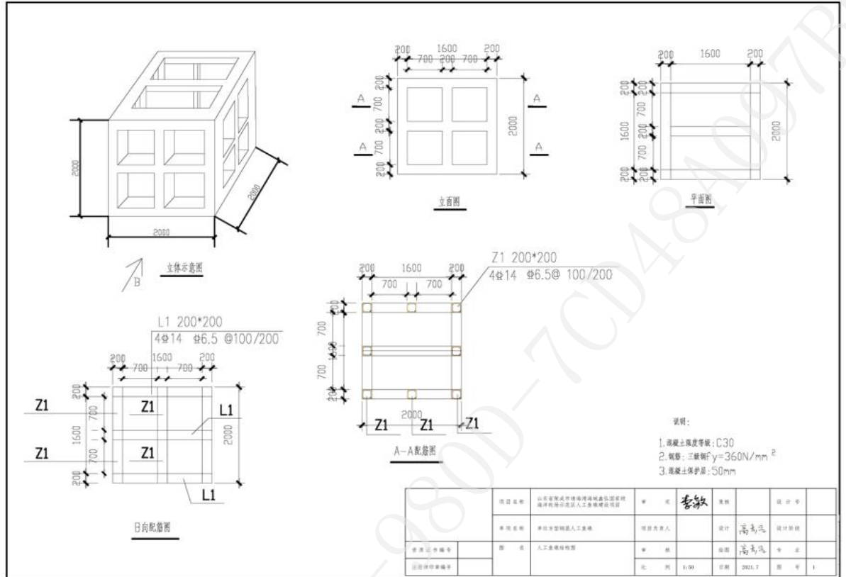
2m 立 方 体 田 字 形 钢 混 构 件 确 示 意 图
