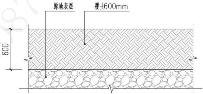
图 5-2 旱地复垦做法详图
