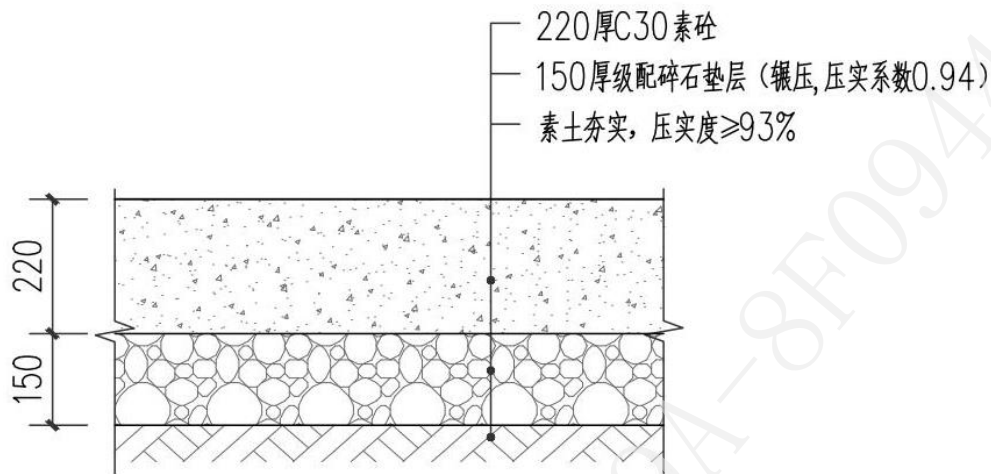
图 5-10 混凝土道路剖面结构示意图
