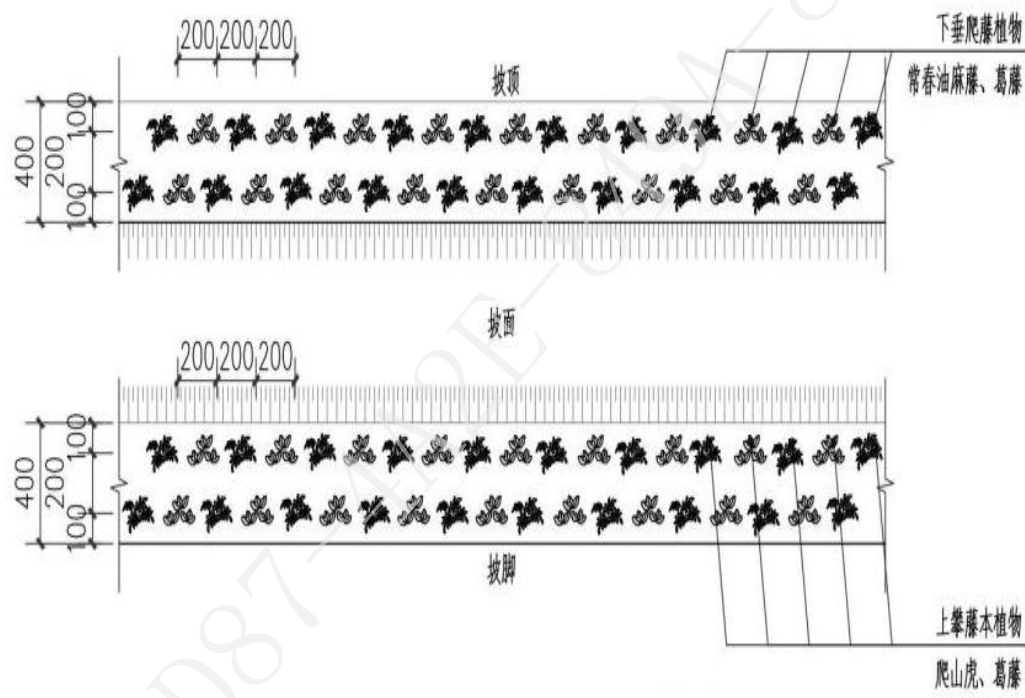
图 5-7 藤本植物种植带平面结构示意图
