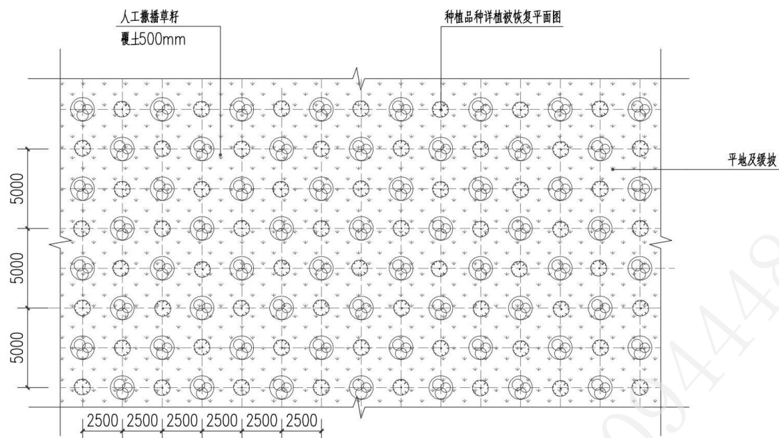
图 5-8 人工种植绿化工艺平面示意图
