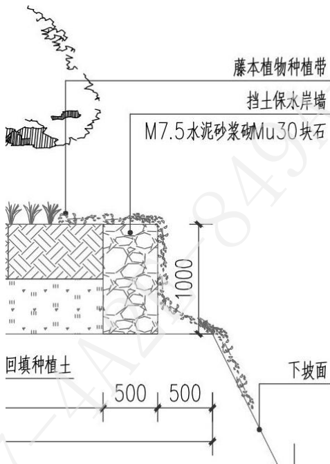
图 5-3 挡土墙剖面结构示意图
