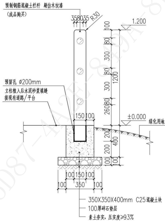
图 5-14 安全护栏侧剖面图
