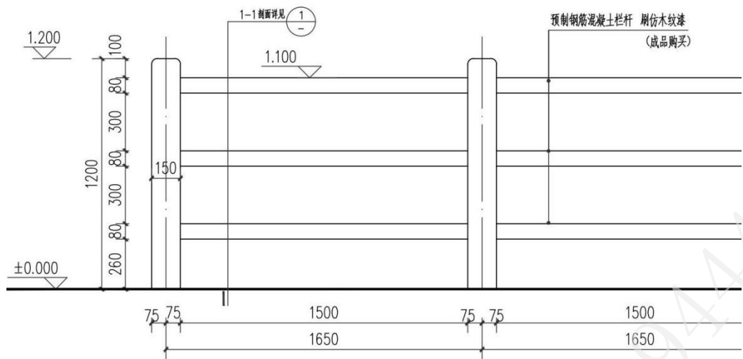
图 5-13 安全护栏立面图
