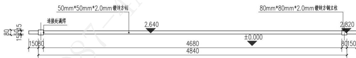
图 5-18 工程简介牌平面图
