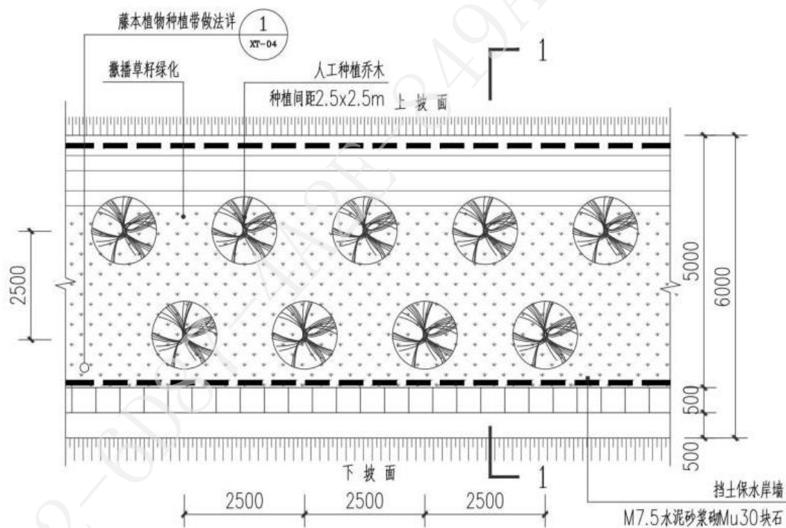
图 5-5 分级平台绿化工艺平面示意图
