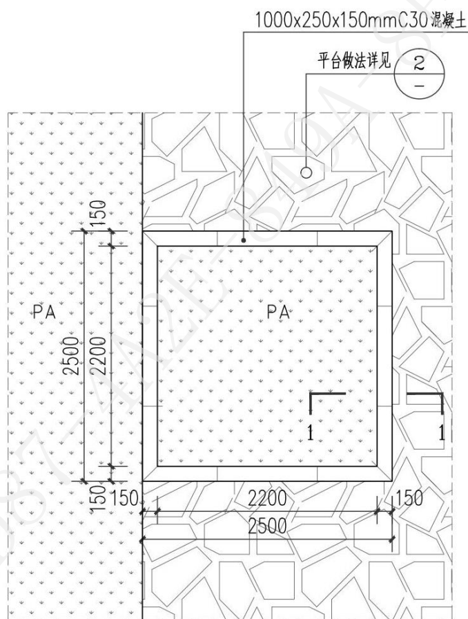
图 5-12 树池平面图
