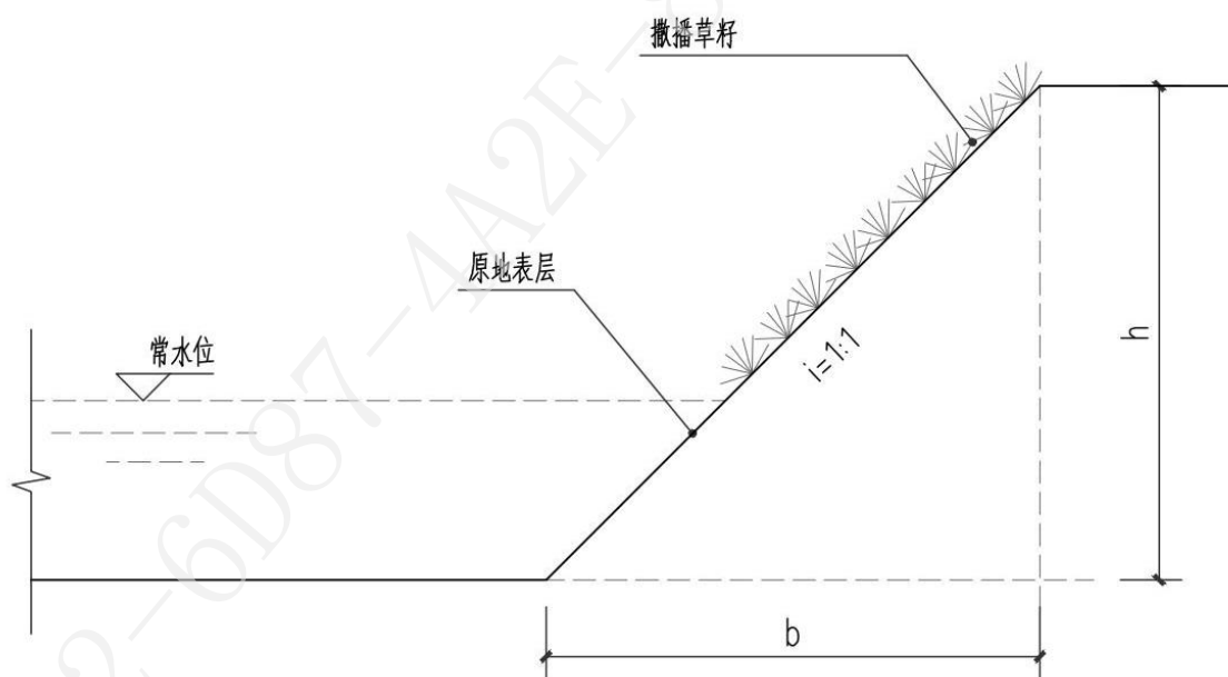
图 5-16 水塘剖面结构示意图
