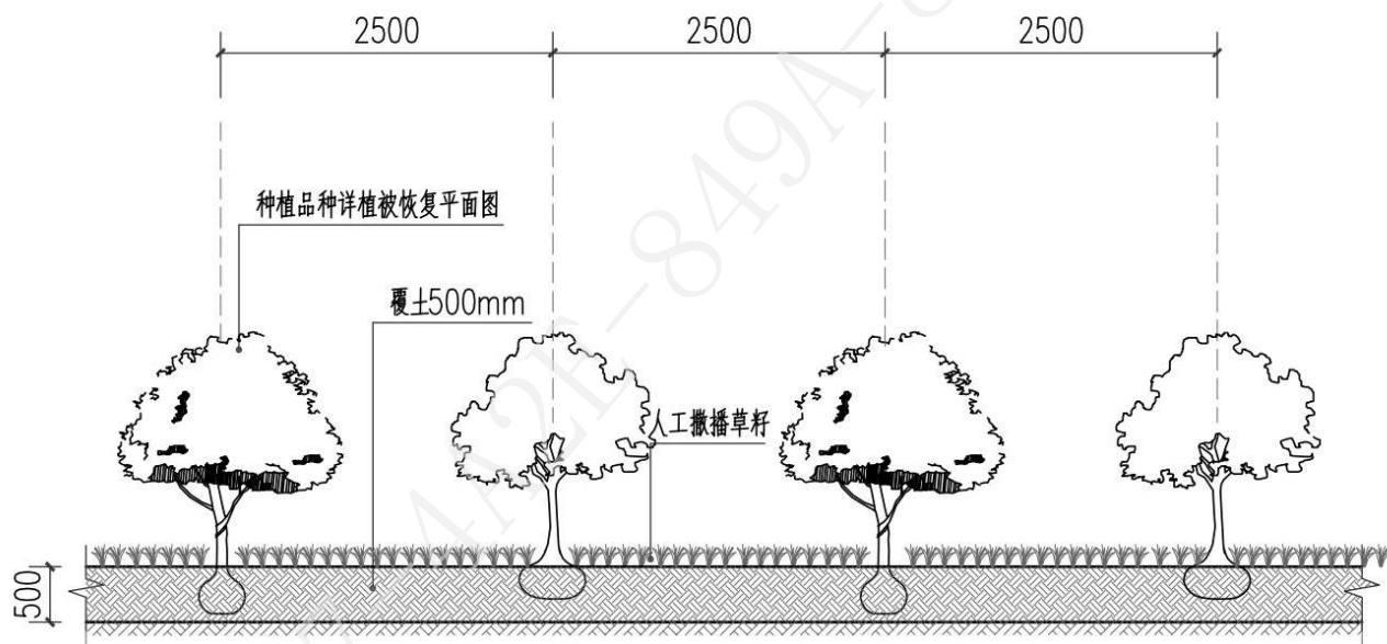
图 5-9 人工种植绿化工艺平地剖面示意图
