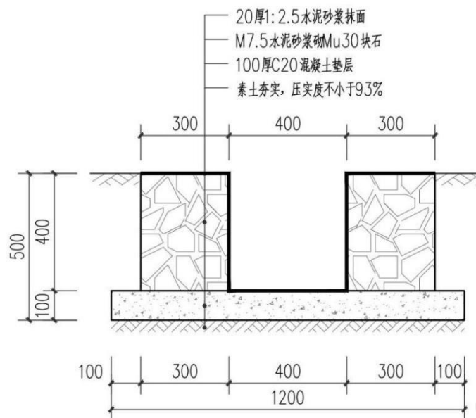
图 5-4 截排水沟剖面结构示意图
