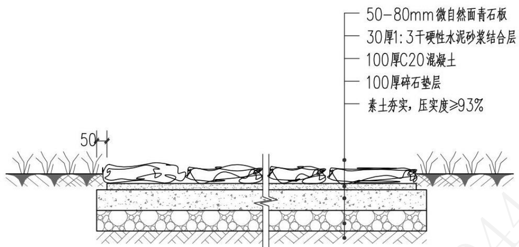
图 5-11 平台/步道剖面图
