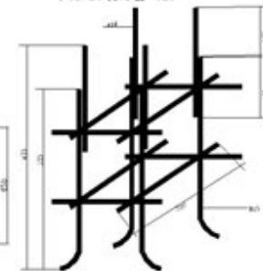
图3 基础预埋件结构示意图
