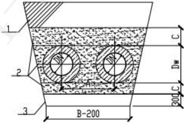
非 cohesion 性黄土，地下水位以下 直埋管道横断面布置图
