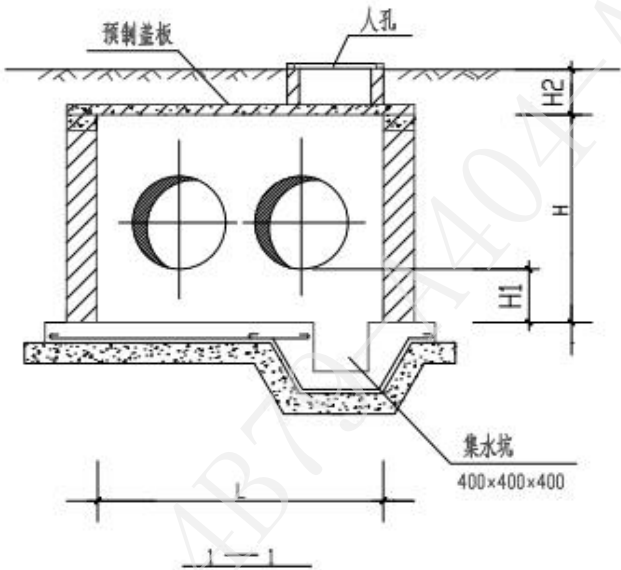
阀门井工艺参考尺寸（保温管道阀门）
