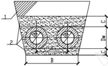
非 cohesion 性黄土，地下水位以上 直埋管道横断面布置图
