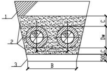
cohesion 性黄土，地下水位以下 直埋管道横断面布置图
