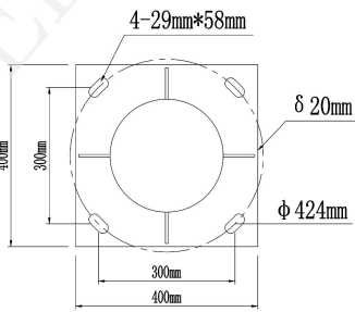
路灯底座法兰盘
