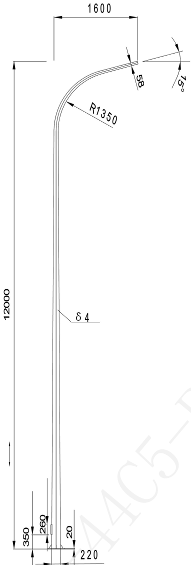
12米单臂路灯灯杆
