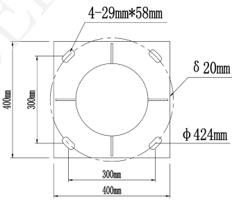
路灯底座法兰盘
