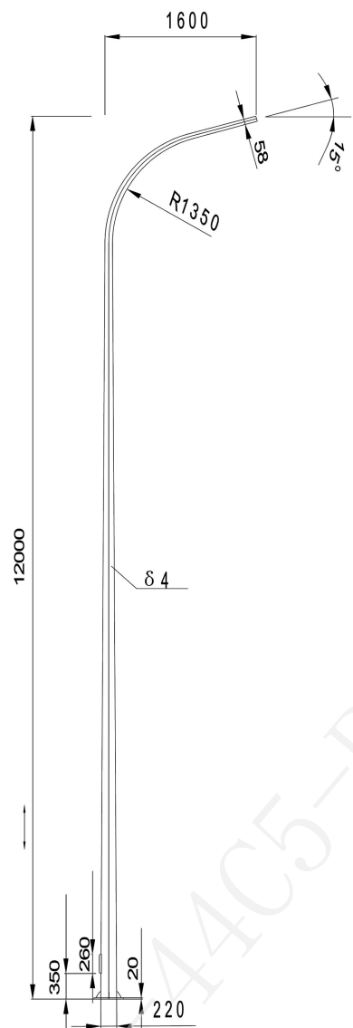
12米单臂路灯灯杆
