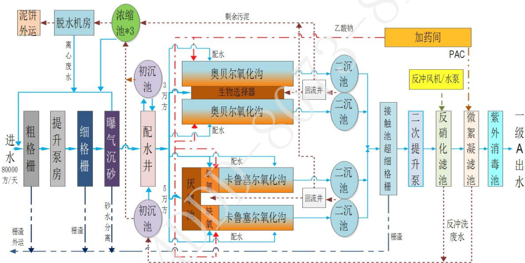
文登污水处理厂工艺流程图
