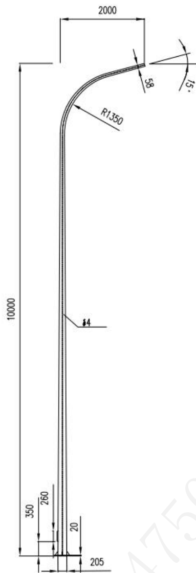
10米单臂路灯灯杆
