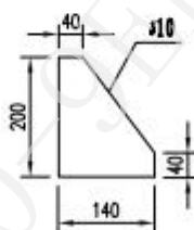
15米中杆灯底部法兰加强筋平面图
