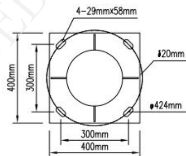
法兰大样图
