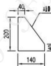
15米中杆灯底部法兰加强筋平面图
