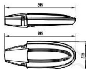
240W灯头尺寸图
