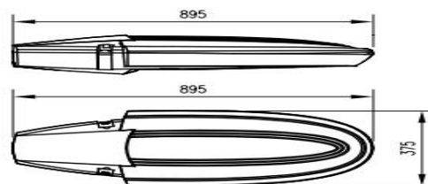
240W灯头尺寸图
