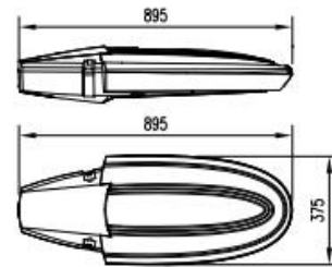
200W灯头尺寸图
