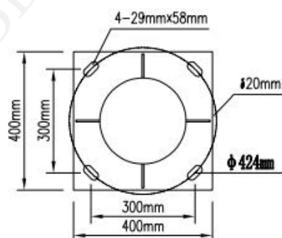
法兰大样图
