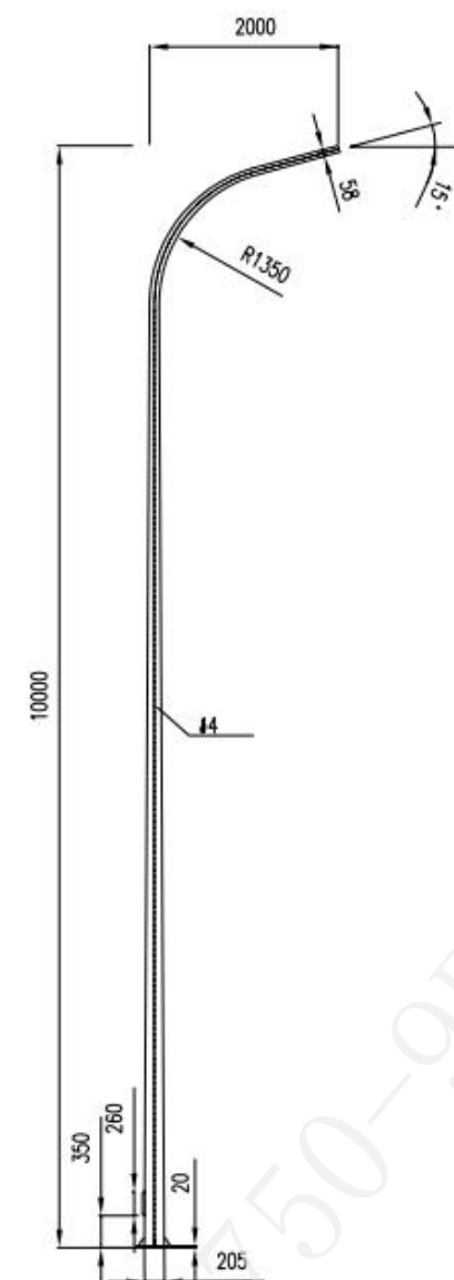
10米单臂路灯灯杆
