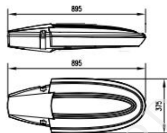
150W灯头尺寸图
