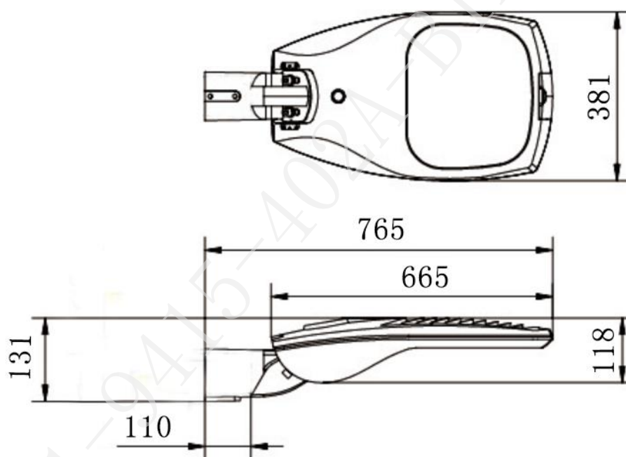
灯头图纸
