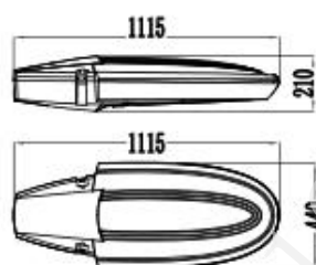
LED灯头240W尺寸图
