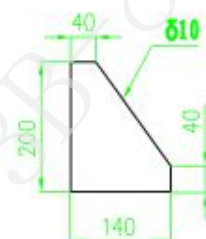
16米中杆灯底部法兰加强筋平面图
