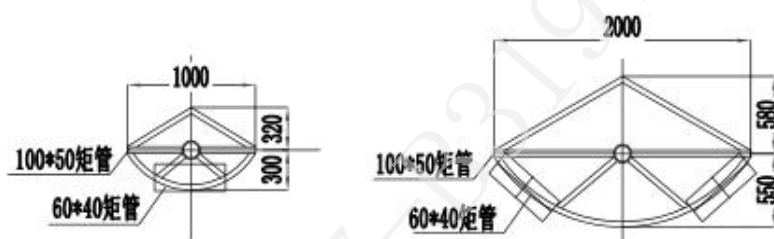
灯盘俯视图
