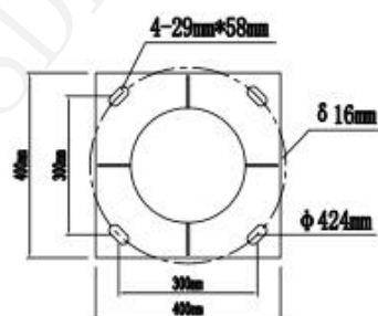
法兰大样图
