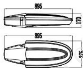
LED灯头240W尺寸图
