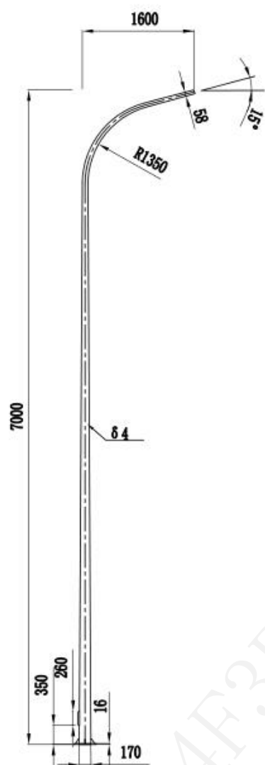
7米单臂路灯灯杆
