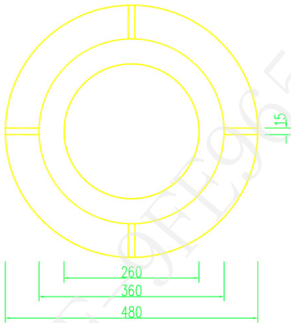
防撞筒平面图
