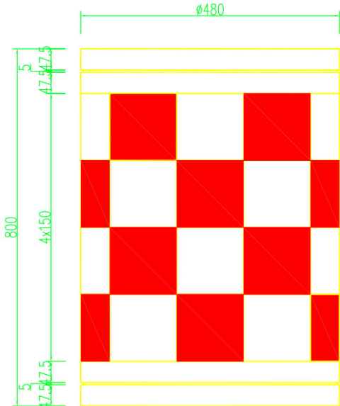
防撞筒立面图
