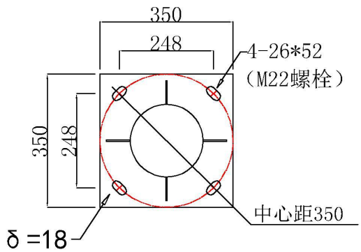
底法兰示意图
