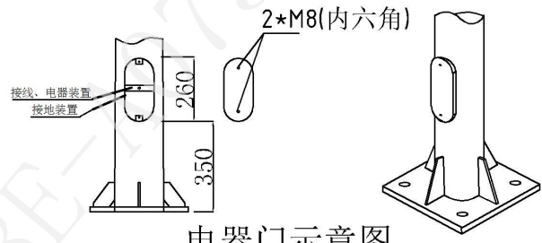
电器门示意图
