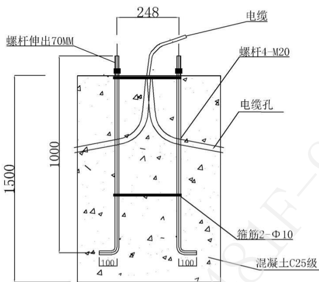
路灯基础
