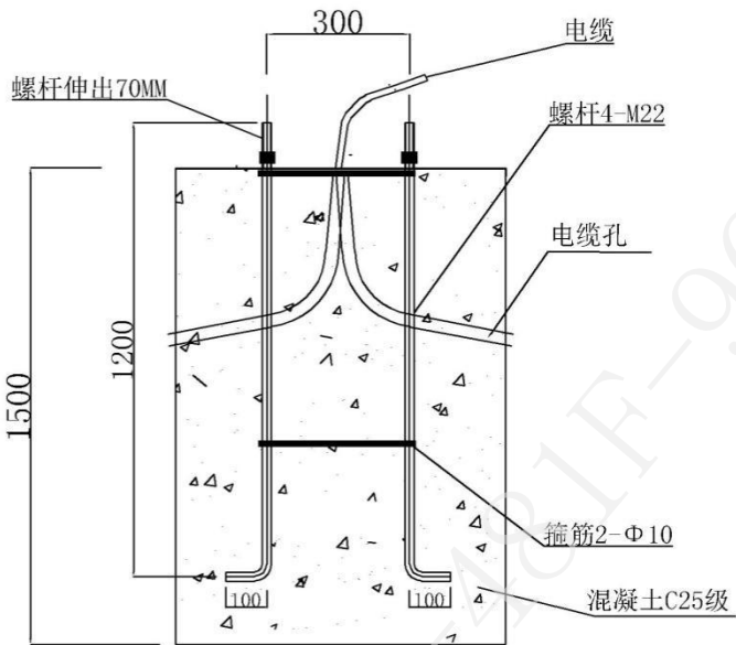
路灯基础
