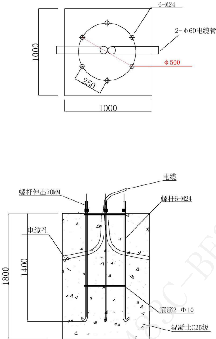
路灯基础
