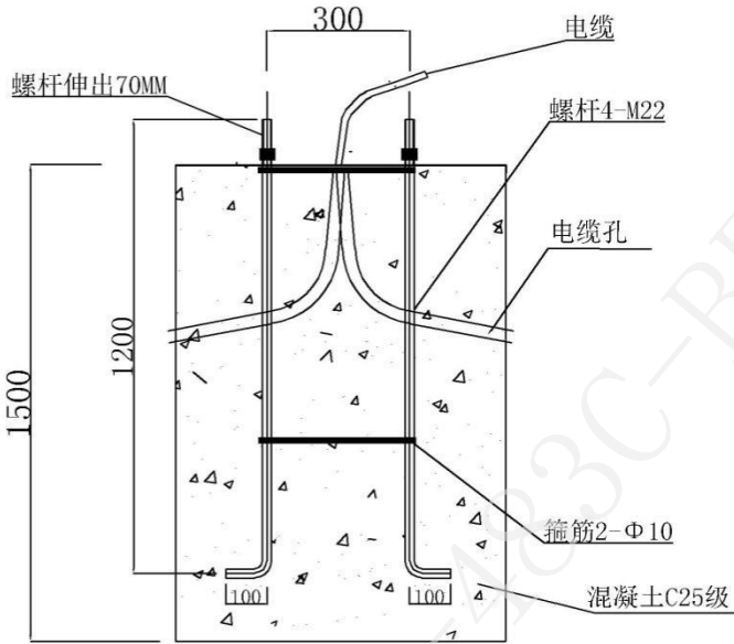
路灯基础
