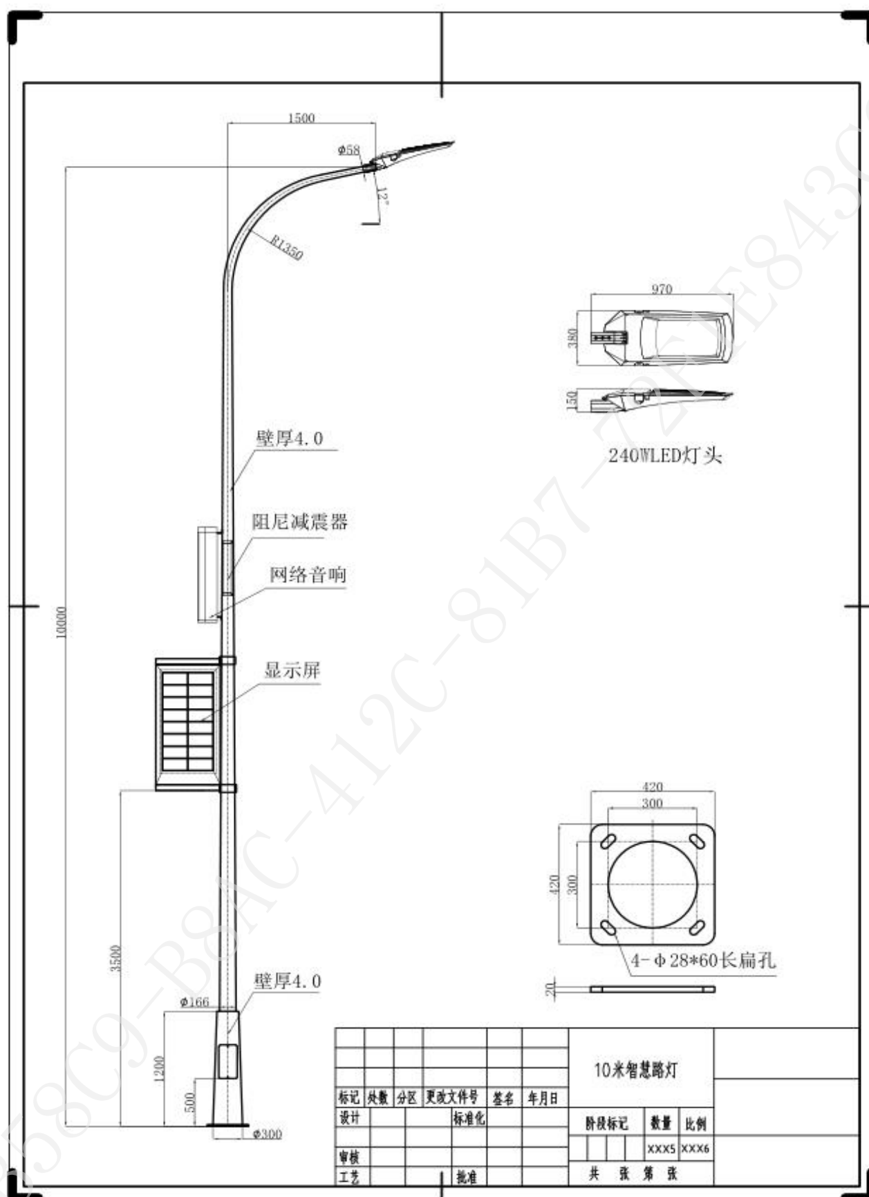
路灯技术图
