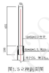
路段式路名牌结构图二
