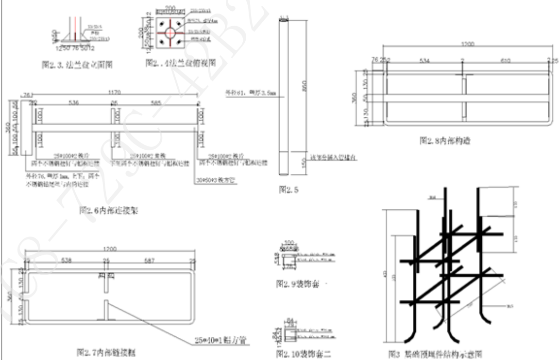
路口式路名牌结构图二
